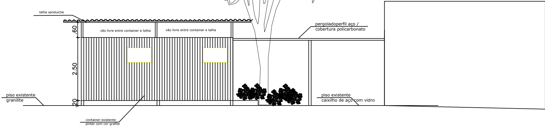
FACHADA REFORMA BANHEIROS
